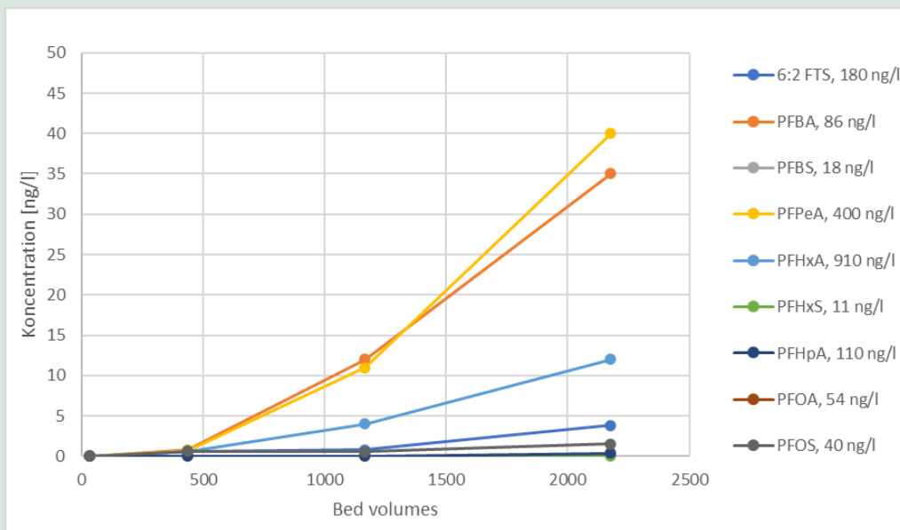
FIGUR 23. PFAS-koncentration i udløbsvandet fra resinkolonner (Purolite PFA694E). Indløbsvand var ubehandlet rejeckt vand fra slambedene. Koncentrationen, der er angivet efter PFAS-navnene, indikerer indløbskoncentrationerne af de forskellige PFAS-stoffer.
