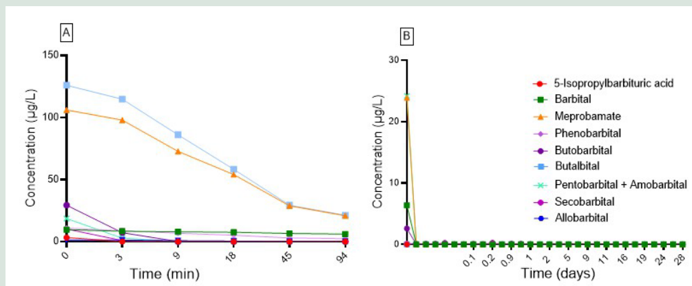
FIGUR 11. Barbiturat resultater fra ozonering (A) og GAC (B) forsøg.
