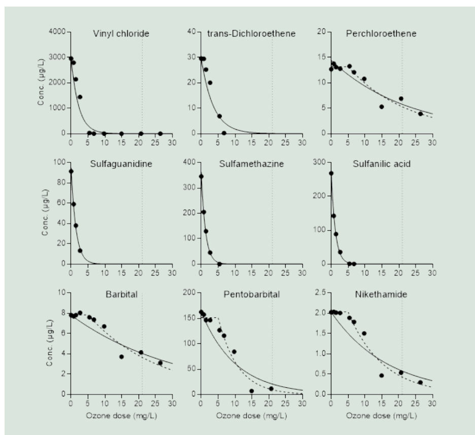
FIGUR 5. Koncentration af 9 forureningsstoffer efter behandling med forskellige ozondoser i en grundvandsprøve udtaget fra område med høj udledning af vinylchlorid til Grindsted Å, hvor det er sandsynligt, at en behandlingsløsning vil blive placeret.
