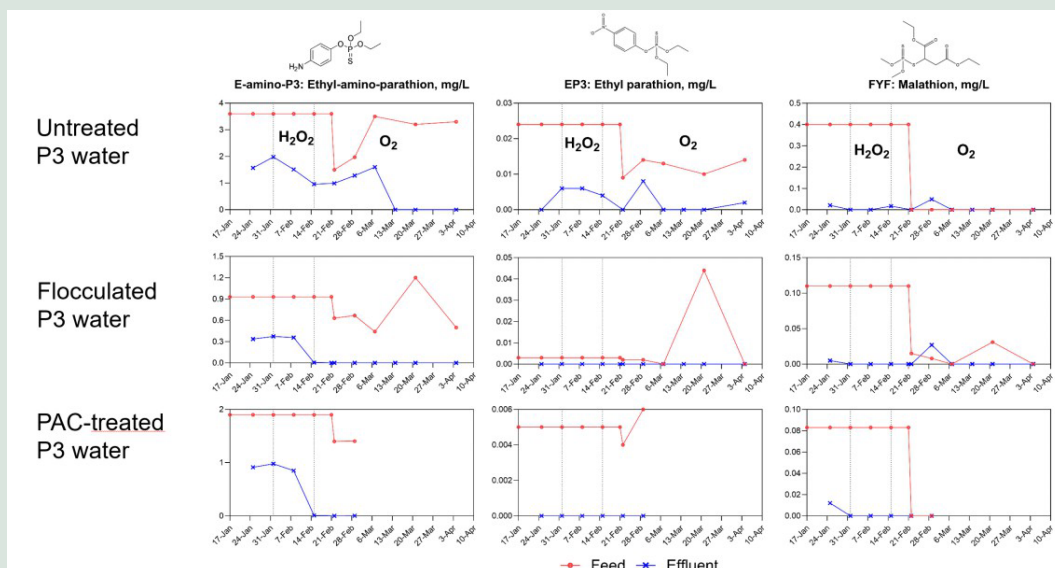
FIGUR 54. Organofosforinsekticiders profil i ubehandlet/forskelligt forbehandlet P3-afværgvand i driftsperioden.
