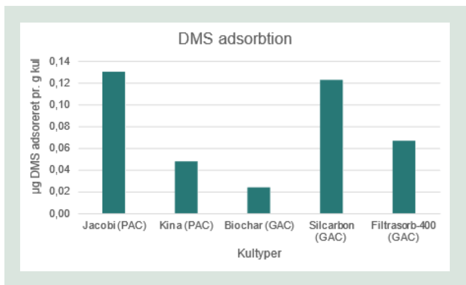
FIGUR 31. Y-aksen: DMS-adsorption pr. g kul ( \mu\text{g/g} ). X-aksen: forskellige kultyper testet under kolbeforsøgene.
