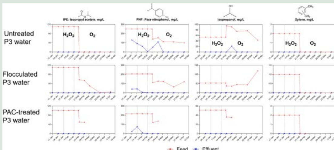
FIGUR 55. Profilen af produktionskemikalier i ubehandlet/ forskelligt forbehandlet P3-afværgvand i driftsperioden.
