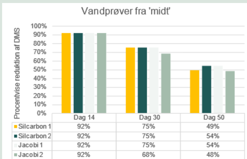
FIGUR 35. Procentvis reduktion af DMS i kolonner fra prøveudtagning 'midt'. For hver type af aktivt kul var der opsat to kolonner. Prøverne her er udtaget midt i filteret. Farverne indikerer dag i forsøgsperioden for udtagelse af vandprøve.
