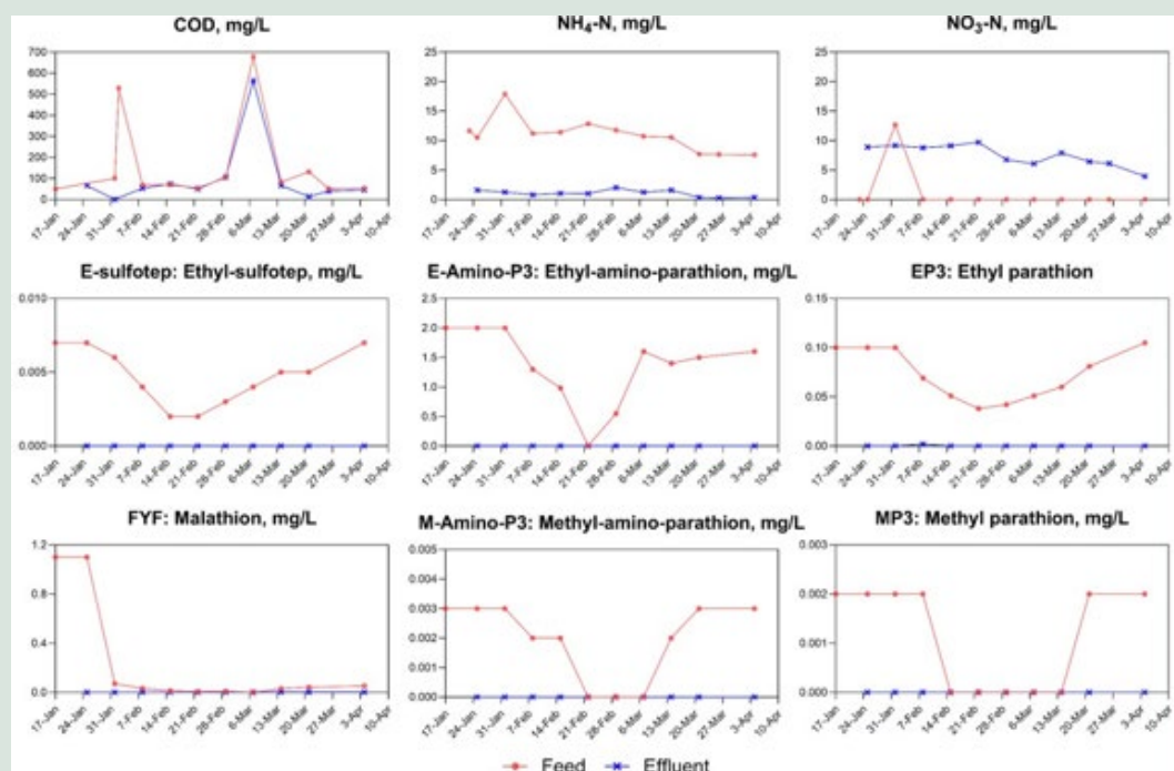
FIGUR 56. Resultater fra GI. fabrik MBBR-pilotforsøg, herunder COD, \text{NH}_4\text{-N} , \text{NO}_3\text{-N} og organofosforinsekticider.
