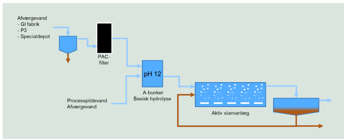
FIGUR 41. Principskitse af det biologiske rensningsanlæg hos FMC-site Rønland.
