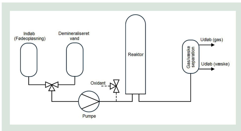
FIGUR 25. Simplificeret procesflowdiagram af Aquarden Technologies' CWO/subCWO-anlæg. Fødeopløsningen, som skal oprenses, tryksættes og blandes med oxidanten (iltberiget luft), hvorefter den opvarmes ved introduktion til den varme reaktor. Oxidation foregår inde i reaktoren, og det behandlede vand forlader systemet gennem en varmeveksler, som sørger for, at reaktionsenergien udnyttes inde i reaktoren, inden vandet gøres trykløst og væske og gas separeres. Der er ikke mekanisk omrøring i reaktoren, men den indre varmeveksler samt luftflowet giver turbulens, hvilket sikrer, at der ikke er nogen stillestående zoner. Anlægget er drevet af elektricitet, og der tilsættes derfor ikke brændsel til opløsninger, som skal destrueres.
