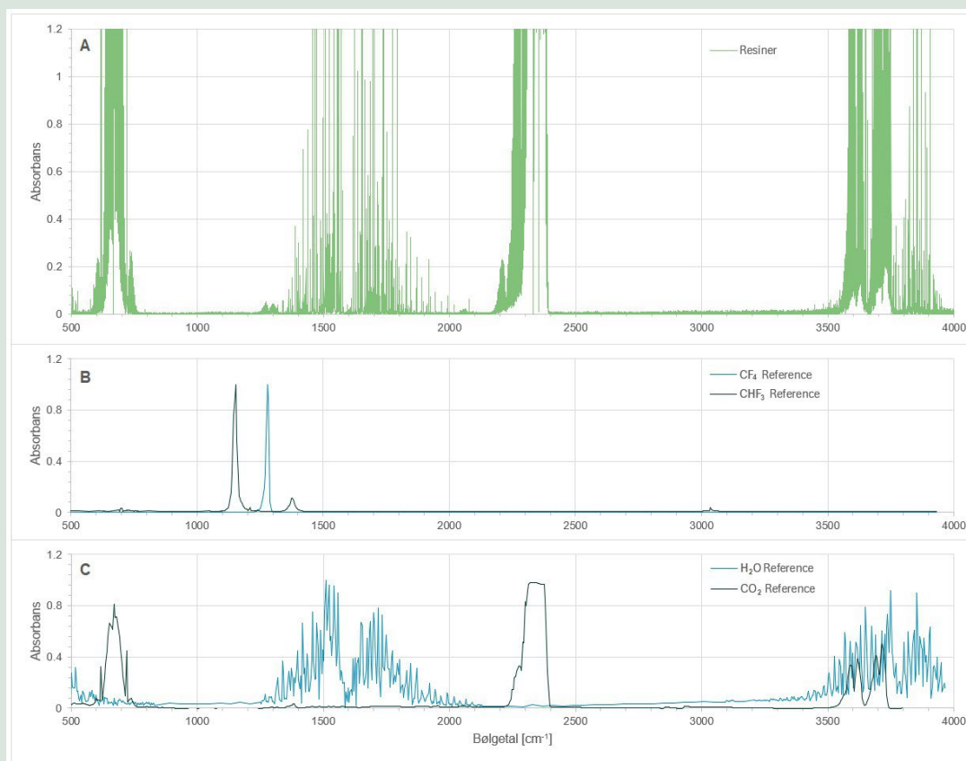
FIGUR 27. IR-spektre til identifikation af gasfaseprodukter for SCWO af resiner fra DIN Forsyning. A) IR-spektrum af udstødningsgassen. B) IR-referencespektre af \text{CF}_4 og \text{CHF}_3 . C) IR-referencespektre af \text{H}_2\text{O} og \text{CO}_2 . Referencespektre er fra den kemiske database udarbejdet af National Institute of Standards and Technology (NIST).
