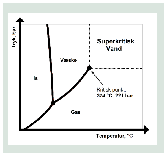
FIGUR 24. Fasediagram for vand inklusive det kritiske punkt.
