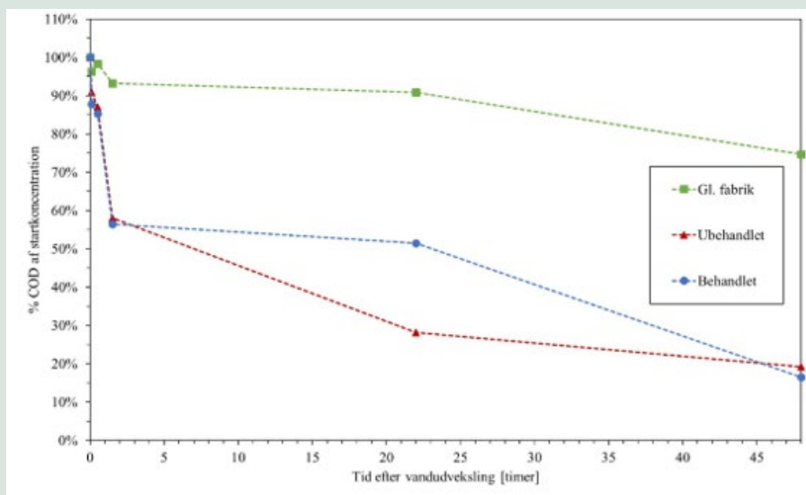
FIGUR 46. Procentvis reduktion af Chemical Oxygen Demand (COD) i MBBR'er, der behandler FMC-vand fra Gl. fabrik, ubehandlet P3-vand og vand fra P3 forbehandlet med 300 mg/L PAC og C/F efter komplet vandudskiftning på dag 54 (100 %).
