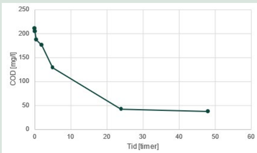
FIGUR 19. COD-omsætning i MBBR med rejeckt vand fra DIN Forsynings slambede tilsat fosfatbuffer.
