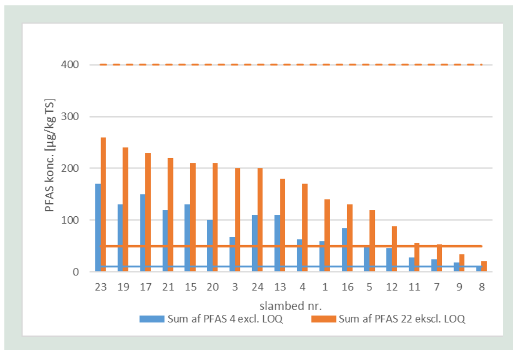
FIGUR 14. PFAS-koncentration i slammet fra slambedene sorteret fra bede med højeste til la-veste koncentration af PFAS. De vandrette linjer indikerer grænseværdierne for slam på 10 µg/kg TS for PFAS sum 4 og 50 µg/kg TS for PFAS sum 22. Den stiplede linje ved 400 µg/kg TS for PFAS sum 22 repræsenterer vejledende grænseværdier for PFAS 22 gældende indtil 30. maj 2024.
