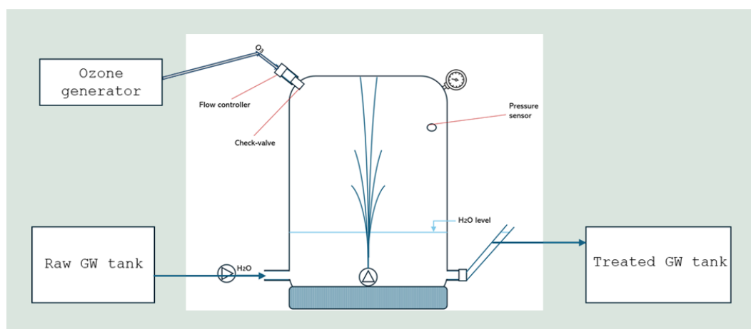
FIGUR 8. Skematisk diagram af den afgasfrie ozoniseringsbehandlingsproces.
