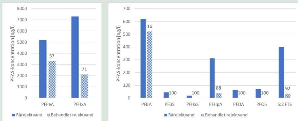
FIGUR 21. PFAS-fjernelse fra rejektvand ved forbehandling. De forskellige PFAS-stoffer i re-je-ktvandet er vist før og efter forbehandlingen med PAX, polymer og Fluorloc efter sett-ling af slammet. Tallene på behandlet rejektvand-kolonnerne indikerer % PFAS-fjernelse. Ved angivelse af 100 % lå værdien under detektionsgrænsen.
