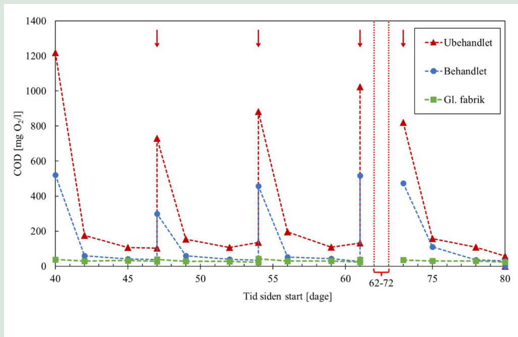
FIGUR 45. Reduktion i COD i MBBR med vand fra Gl. fabrik, P3 ubehandlet og P3 forbehandlet (300 mg/l PAC + koagulering/flokkulering). Vandet havde en opholdstid på 1 uge. Dage 62-72 er grafisk sammenpressede, da der ikke blev udskiftet vand i denne periode.
