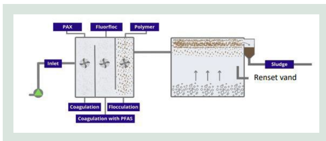
FIGUR 30. Illustration af renseløsning til PFAS-fjernelse fra slambet-rejektvand.
