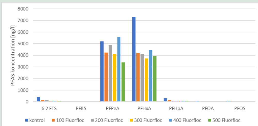
FIGUR 20. Tilsætning af forskellige Fluorloc-koncentrationer til PAX- og polymerforbehandlet rejeckt vand fra slambedene for at finde den optimale Fluorloc-koncentration til fjernelse af PFAS.
