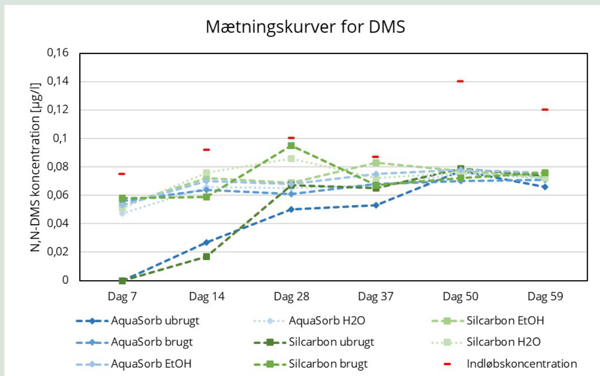
FIGUR 38. Mætningskurver for DMS-koncentration [ \mu\text{g/L} ] over tid for AquaSorb og Silcarbon, både ubrugte, brugte og regenererede med enten ethanol (EtOH) eller vand ( \text{H}_2\text{O} ). Indløbskoncentrationen er angivet som reference.
