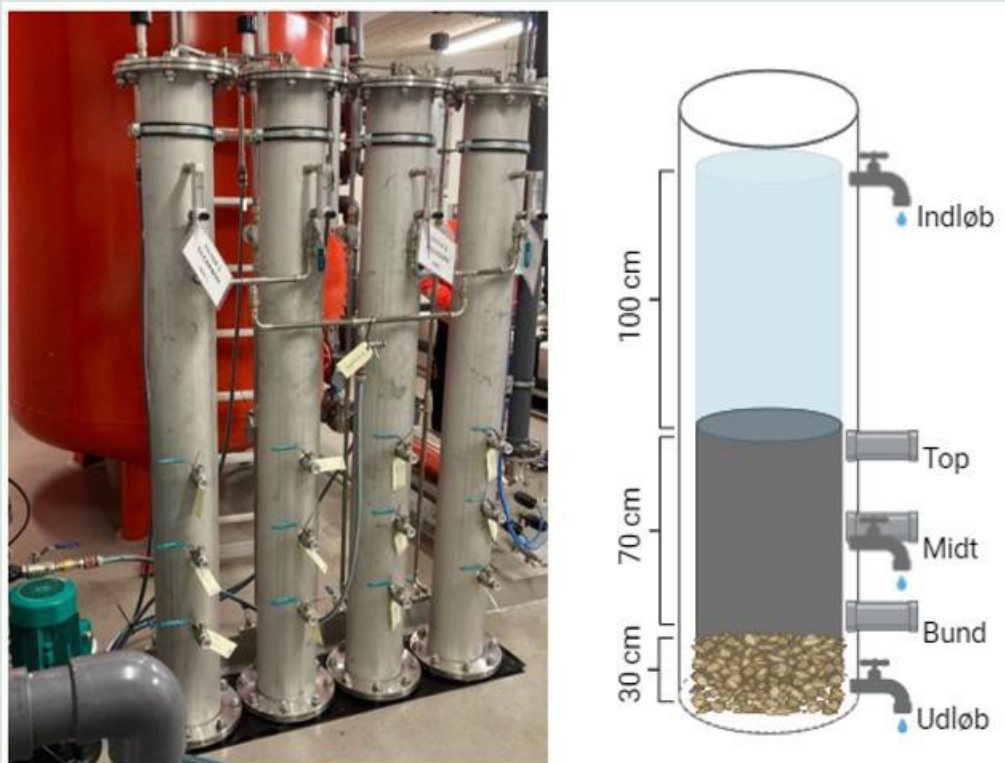
FIGUR 34. Venstre: Tryksatte kolonner på Ærø. To kolonner blev kørt med Silcarbon (GAC), og to kolonner blev kørt med Aquasorb CS (GAC). Højre: Skitse af kolonnerne indefra (fra toppen: 100 cm vand, 70 cm aktivt kul og 30 cm grus). Tappehaner og rør indikerer prøvetagningssteder for hhv. vand (indløb, midt og udløb) og aktivt kul (top, midt og bund).
