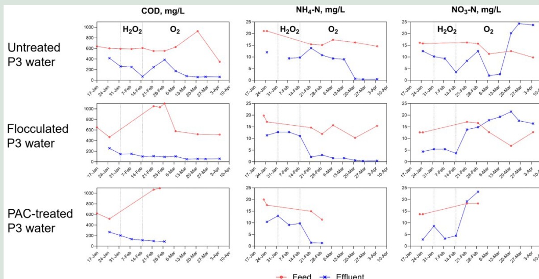
FIGUR 53. COD, ammonium og nitrat i ubehandlet/forskelligt behandlet P3-afværgvand i driftsperioden.
