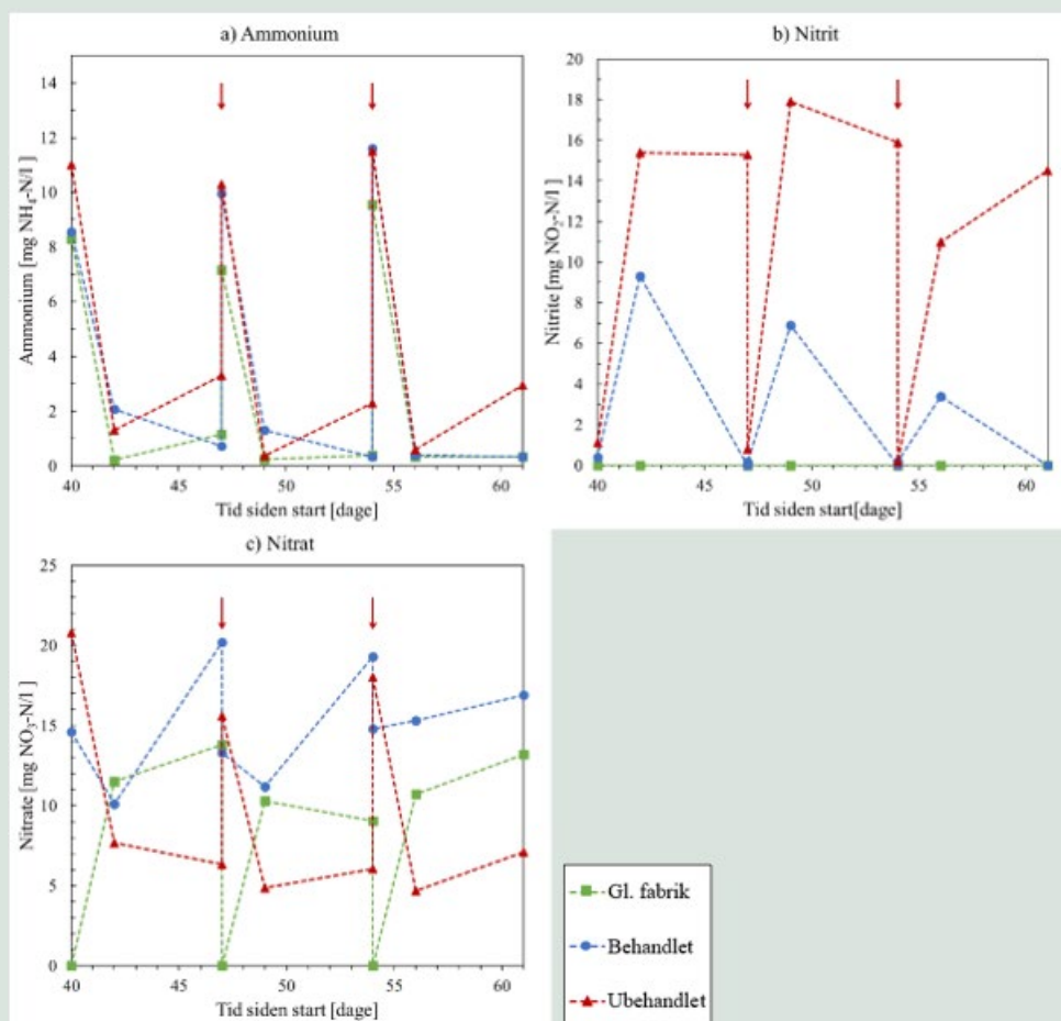
FIGUR 48. Ammonium-, nitrit-, og nitrat-nitrogen-koncentrationer i perioden dag 40-61 i MBBR med vand fra Gl. fabrik, P3 ubehandlet og P3 forbehandlet (300 mg/L PAC + koagulering/flokkulering). Vandet havde en opholdstid på 1 uge.
