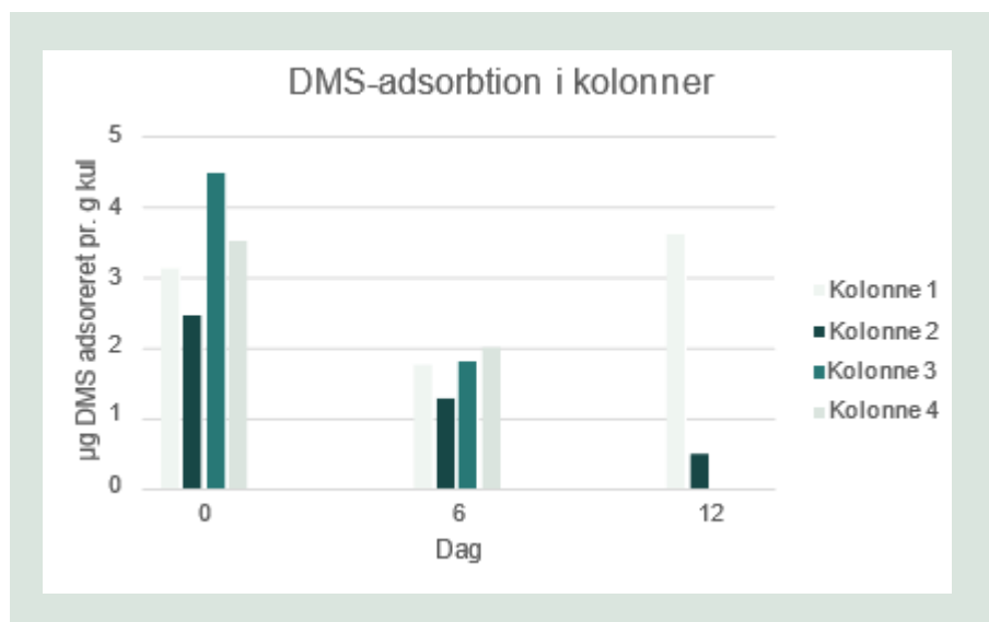
FIGUR 33. Y-akse: \mu\text{g} DMS adsorberet pr. g. kul. X-akse: dag under forsøgsperioden. Farverne indikerer de to kolonner anvendt som replikater. Kolonne 1 og 2 er kørt med Silcarbon. Ses der bort fra dag 12 ved kolonne 1, falder mængden af adsorberet DMS hen over forsøgsperioden. Kolonne 3 og 4 er kørt med Aquasorb CS og ved dag 12 var indløbskoncentrationen meget høj ( 280 \mu\text{g/L} DMS), hvilket resulterede i en urealistisk høj adsorption og resultater er derfor udeladt på grafen.
