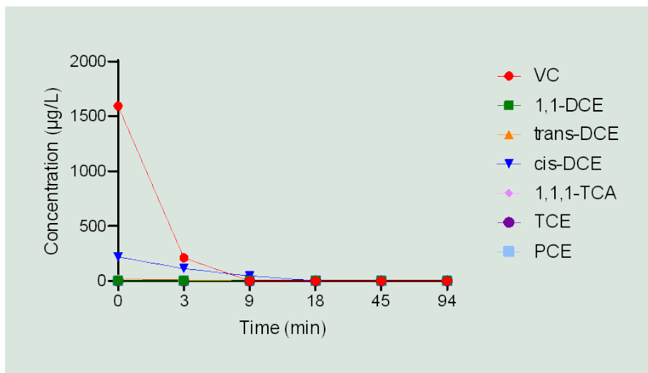
FIGUR 9. Koncentration af chlorerede opløsningsmidler analyseret fra Grindsteds grundvand under pilotforsøget med ozon. Den teoretiske leverede ozon-dosis var 23,7 mg/l.
