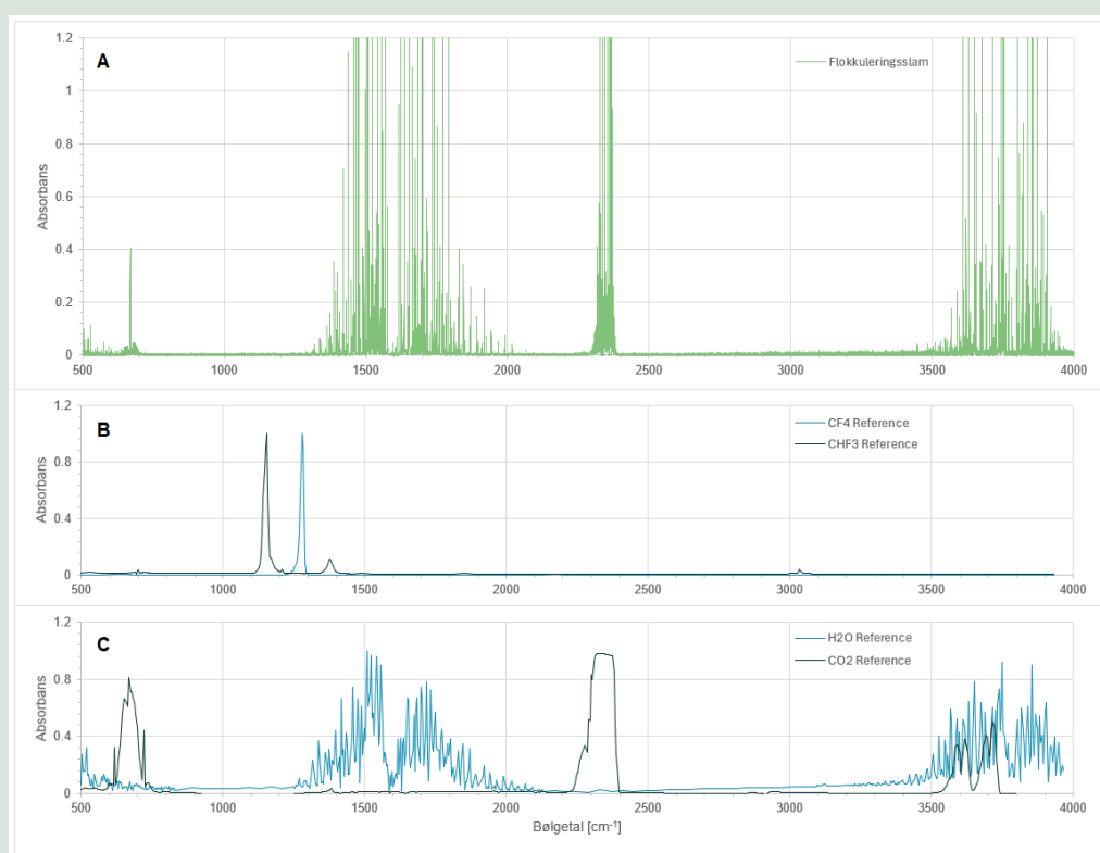
FIGUR 29. IR-spektre til identifikation af gasfaseprodukter fra subCWO af flokkuleringsslam fra DIN Forsyning. A) IR-spektrum af udstødningsgassen. B) IR-referencespektre af CF 4 og CHF 3 . C) IR-referencespektre af H 2 O og CO 2 . Referencespektre er fra den kemiske database udarbejdet af National Institute of Standards and Technology (NIST).
