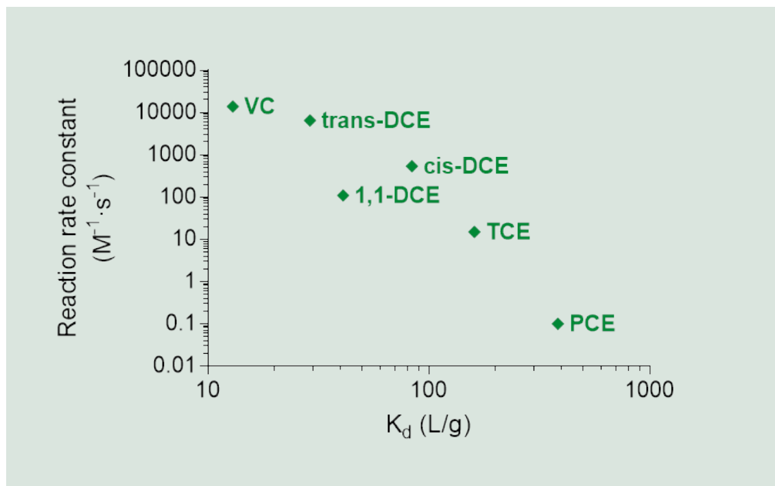
FIGUR 4. Reaktionshastighedskonstant med ozon- og K_d -værdier for forurenende stoffer til stede i Grindsteds grundvand (Kokkoli, Agerholm, Andersen, & Kaarsholm, 2021).
