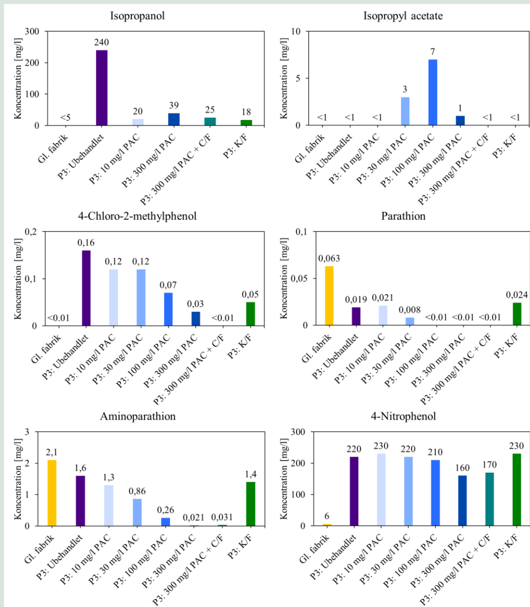
FIGUR 43. Målte koncentrationer af pesticider (parathion, aminoparathion og 4-nitrophenol) og solventer (isopropanol, isopropyl acetat og 4-chloro-2-methylphenol) i afværgvand fra Gl. fabrik, FMC P3 ubehandlet og P3 forbehandlet (300 mg/L PAC + koagulering/flokkulering). Alle kemikalier blev målt af FMC.
