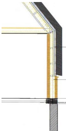
Fig 16. Tværnsnit, Lyngballevej 32, (fra byggesag)
