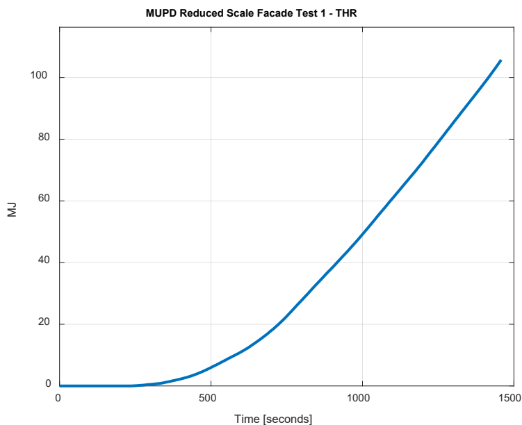
Figur 12. Total Heat Release (THR)
