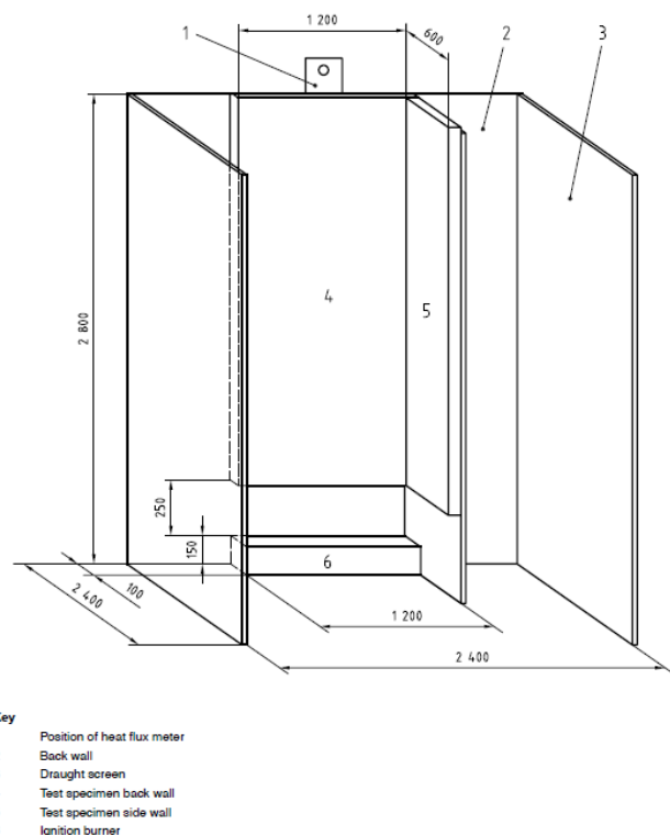
Figur 9. Skaleret facaderig iht. ISO 13785-1
