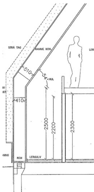
Fig 17. Tværnsnit, Haslevvej 79, (fra byggesag)
