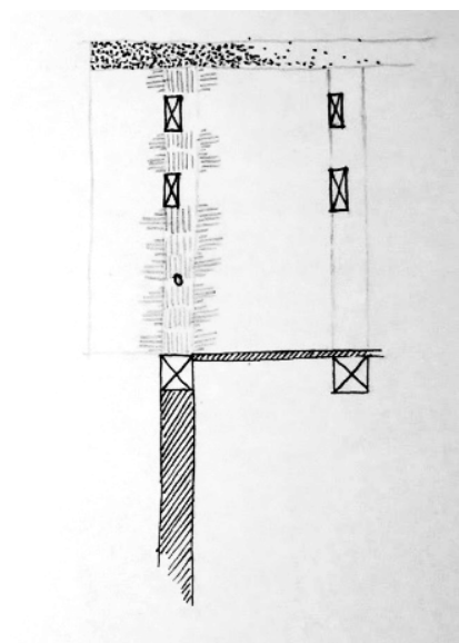
Fig 11. Snit i dukket gavl (HE 2021)
