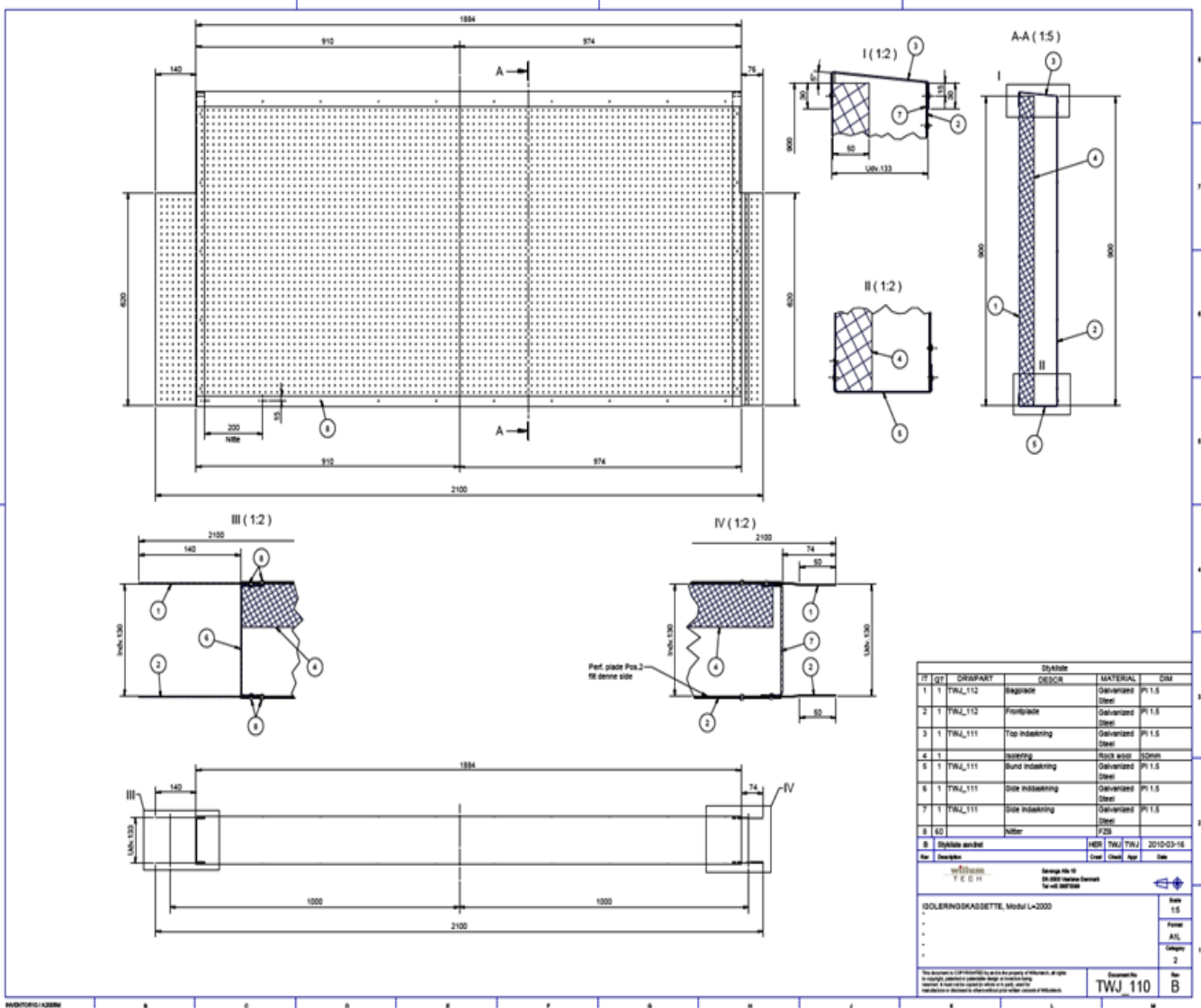
Figur 6. Støjdæmpende sandwichpaneler
