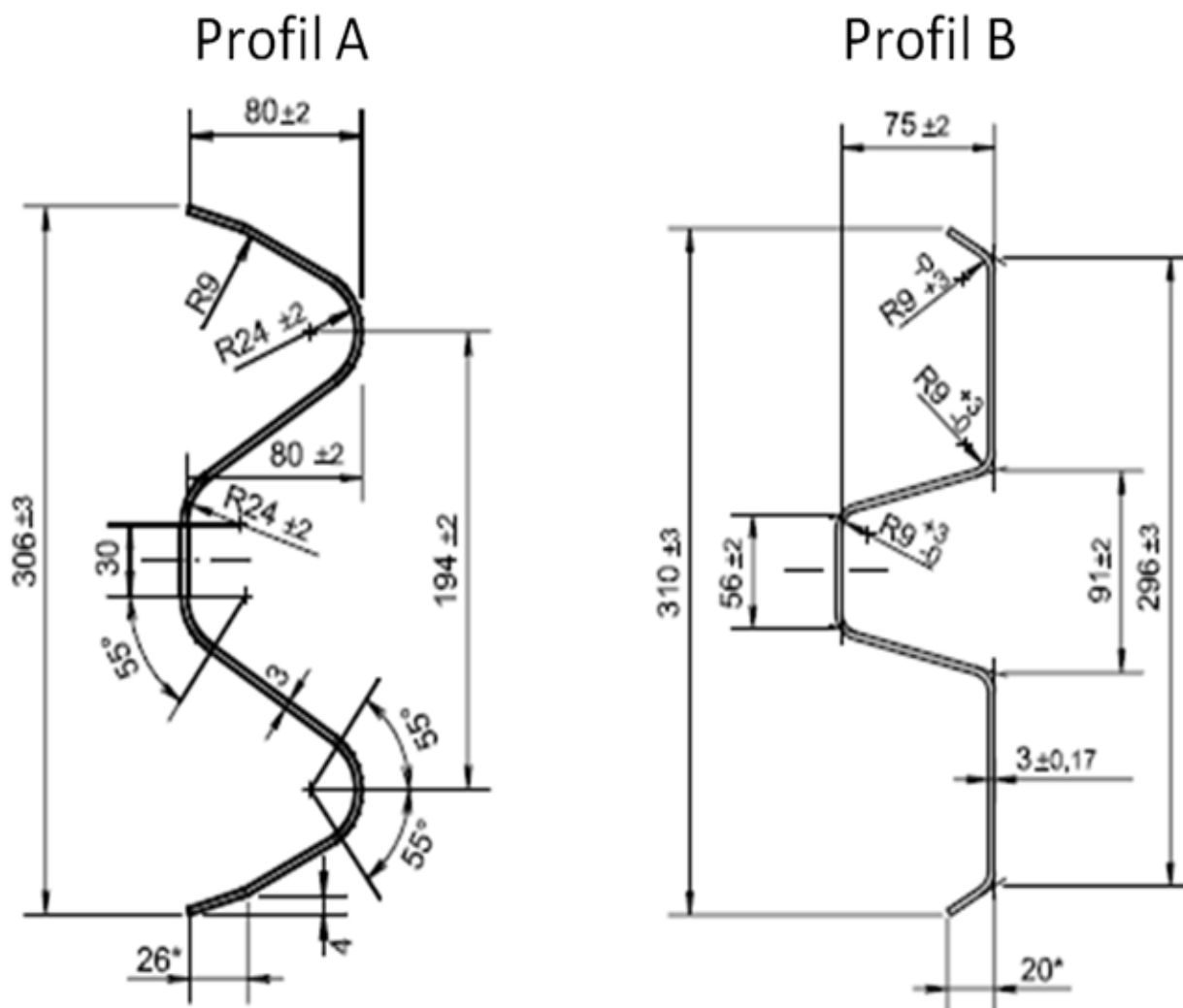
Figur 3. Autoværn profil A og B
