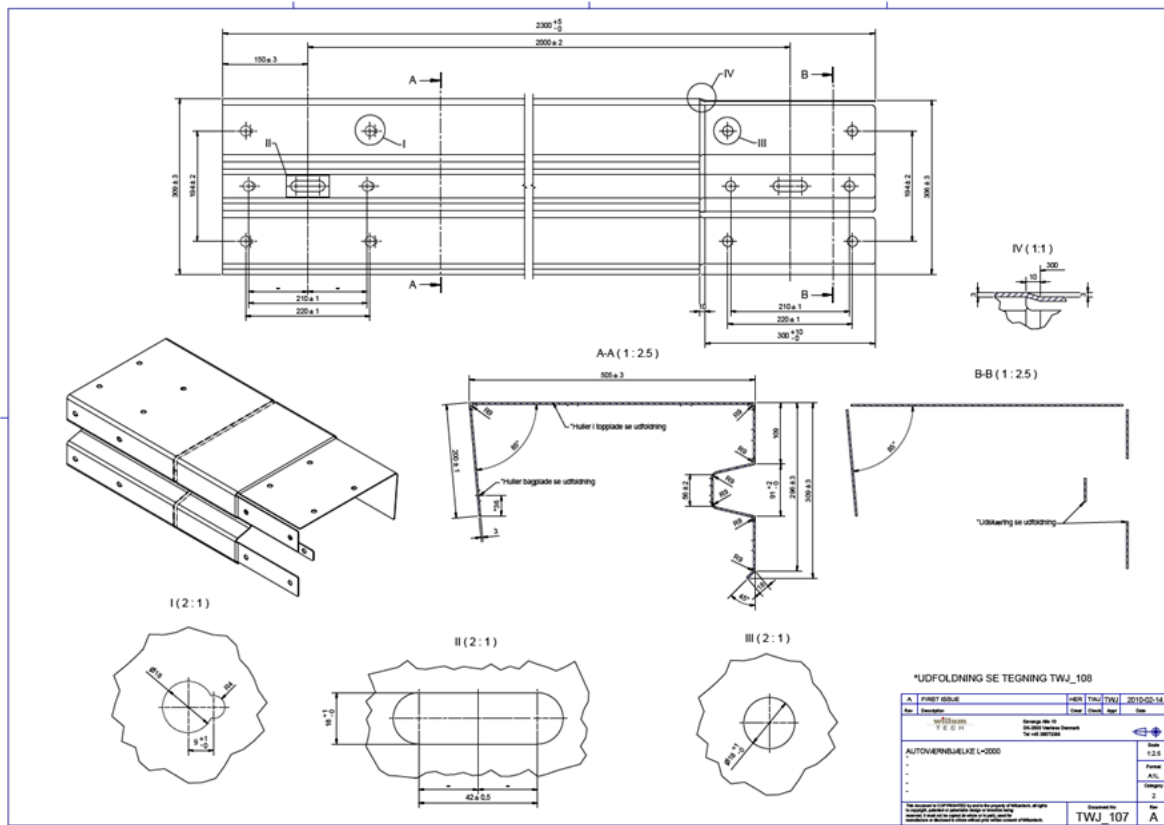
Figur 4. Først blev autoværns bjælken designet
